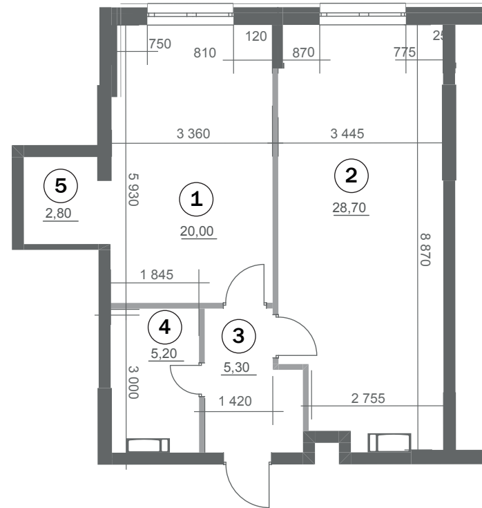
Планування квартири
