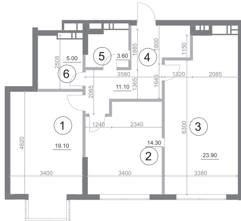
Планування квартири з розмірами
