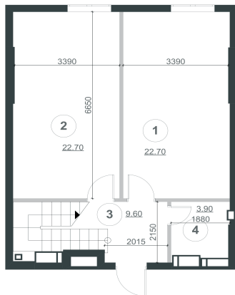
Планування квартири з розмірами
