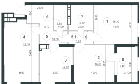
Планування квартири з розмірами
