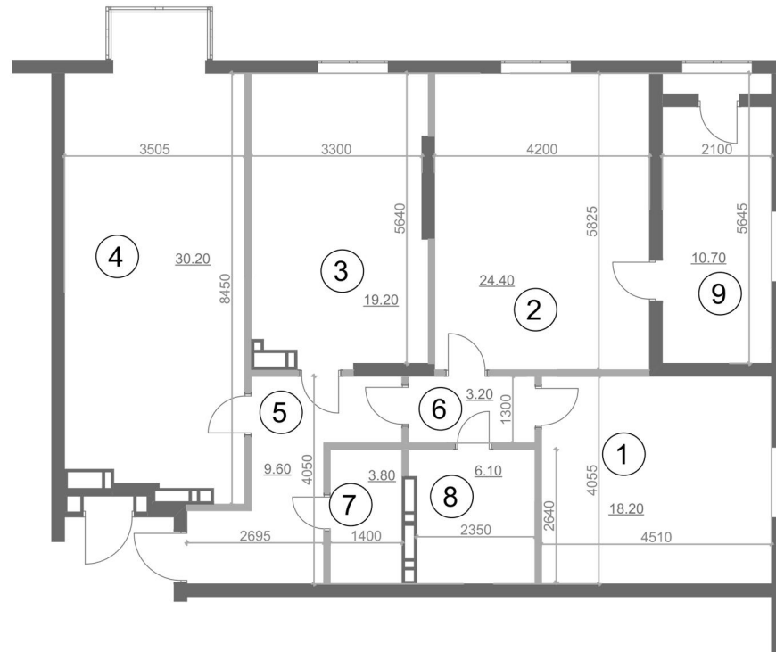
Планування квартири з розмірами
