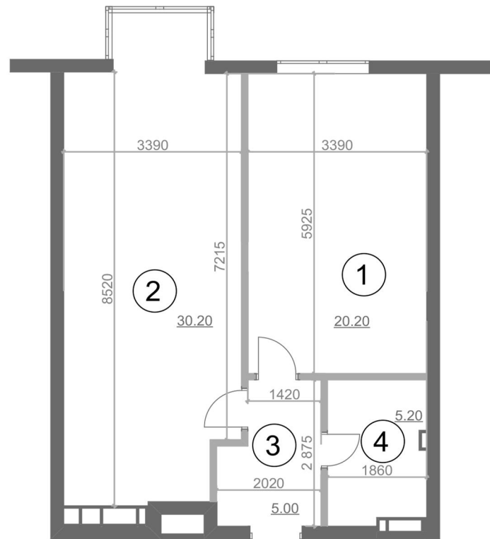
Планування квартири з розмірами
