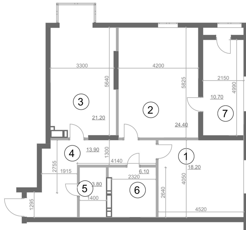
Планування квартири з розмірами
